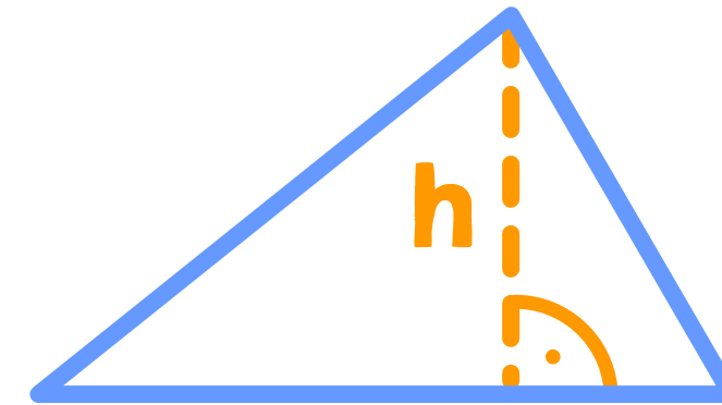
Trójkąt ostrokątny
