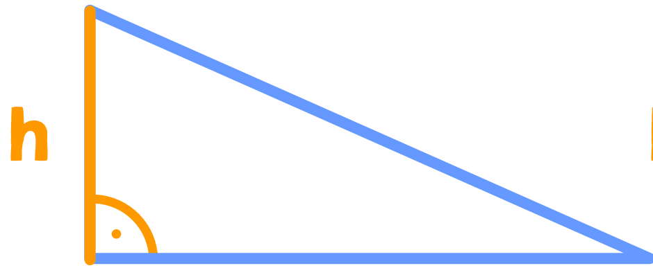
Trójkąt prostokątny
