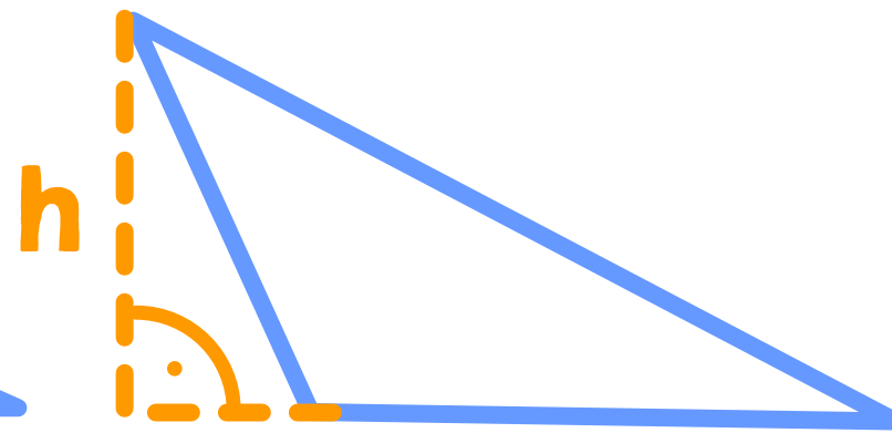
Trójkąt rozwartokątny
