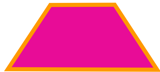
trapez równoramienny
